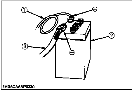
(1) Kalın kırmızı kablo (+)
