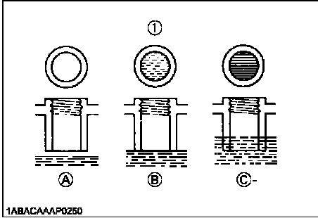
(1) Akü elektrolit seviyesi
